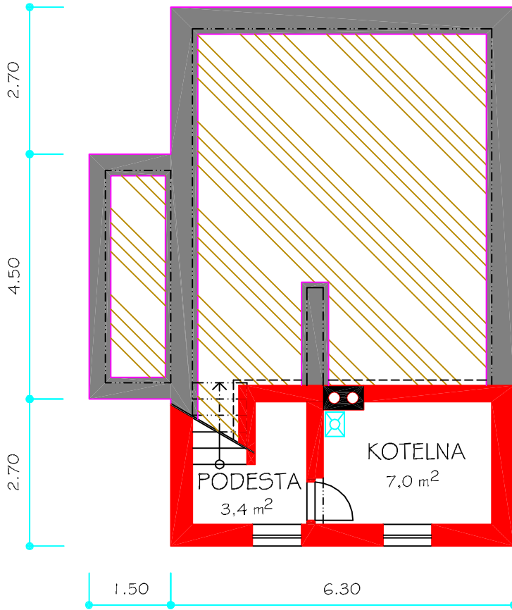
PŮDORYS 1.PP suterén
