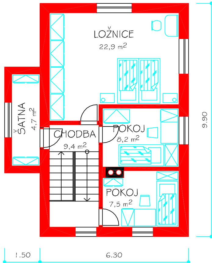
PŮDORYS 2.NP patro
