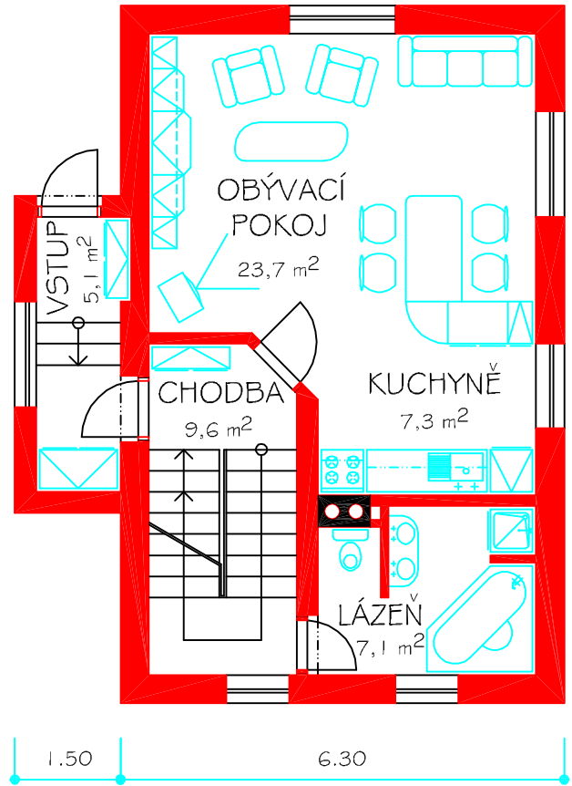
PŮDORYS 1.NP přízemí
